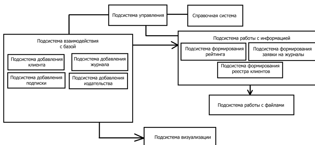
Рис.13 – Структура подпрограмм
